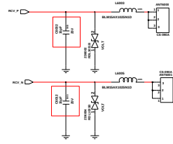
RCV Contact
